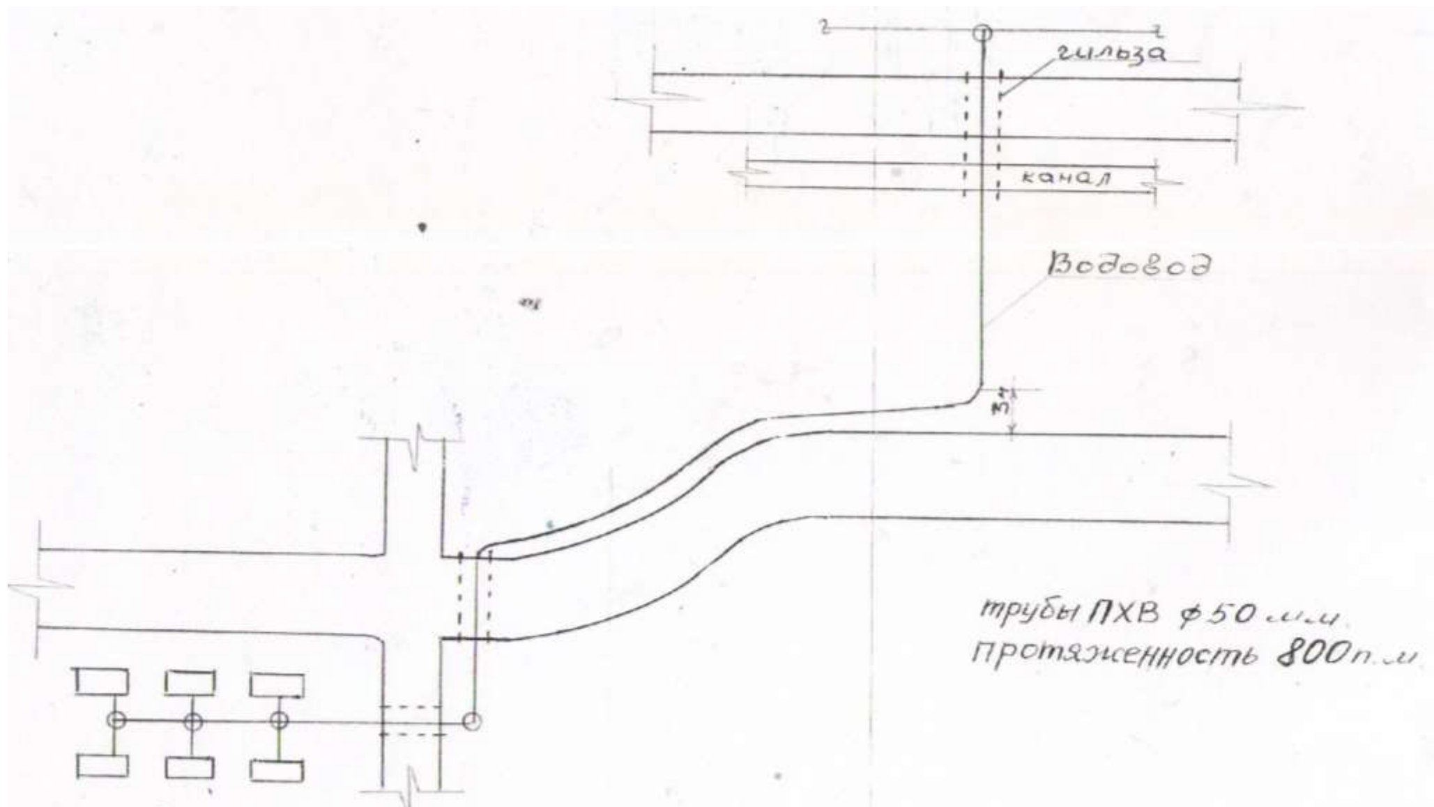
Схема водоснабжения в МКРстадиона «Хазар» для ГУ «МЖП»
