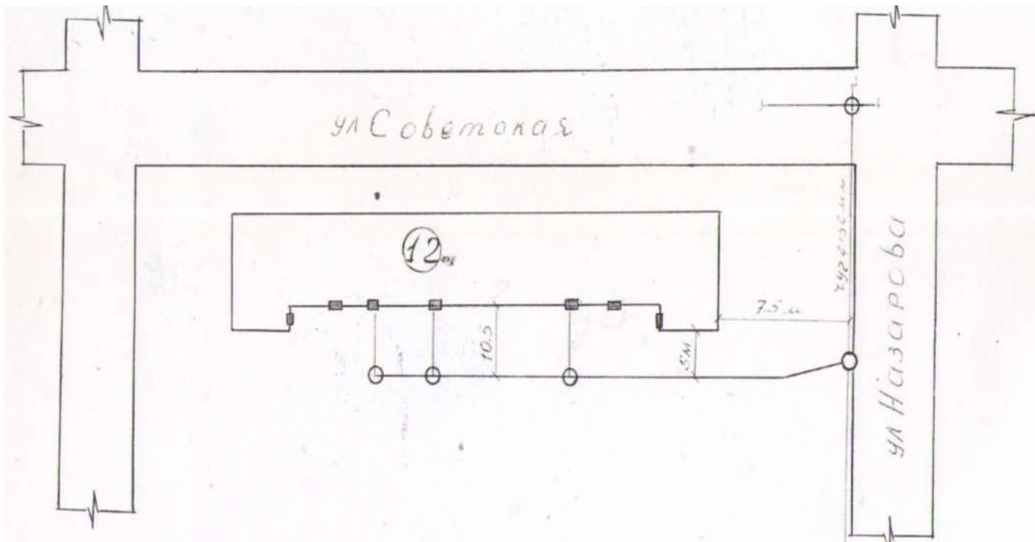
Схема водоснабжения улица Советская 12
