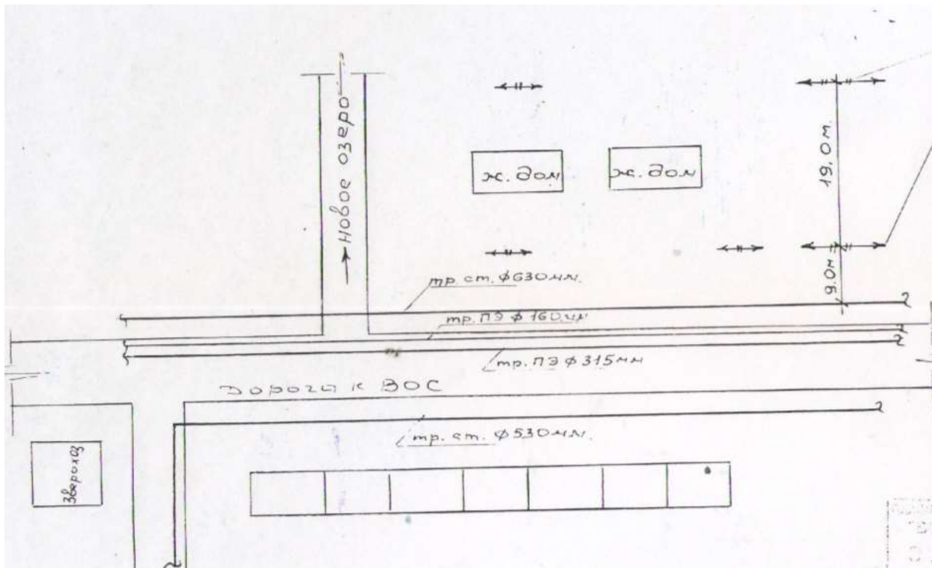
Схема водоснабжения в районе с/о Заря
