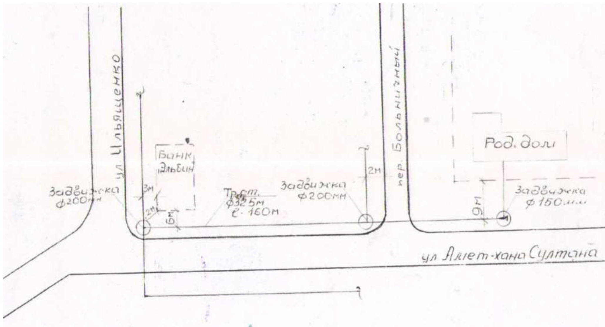
Схема водоснабжения к зданию родильного дома от колодца на пересечении ул. Ильященко и ул. Амет-хана Султана
