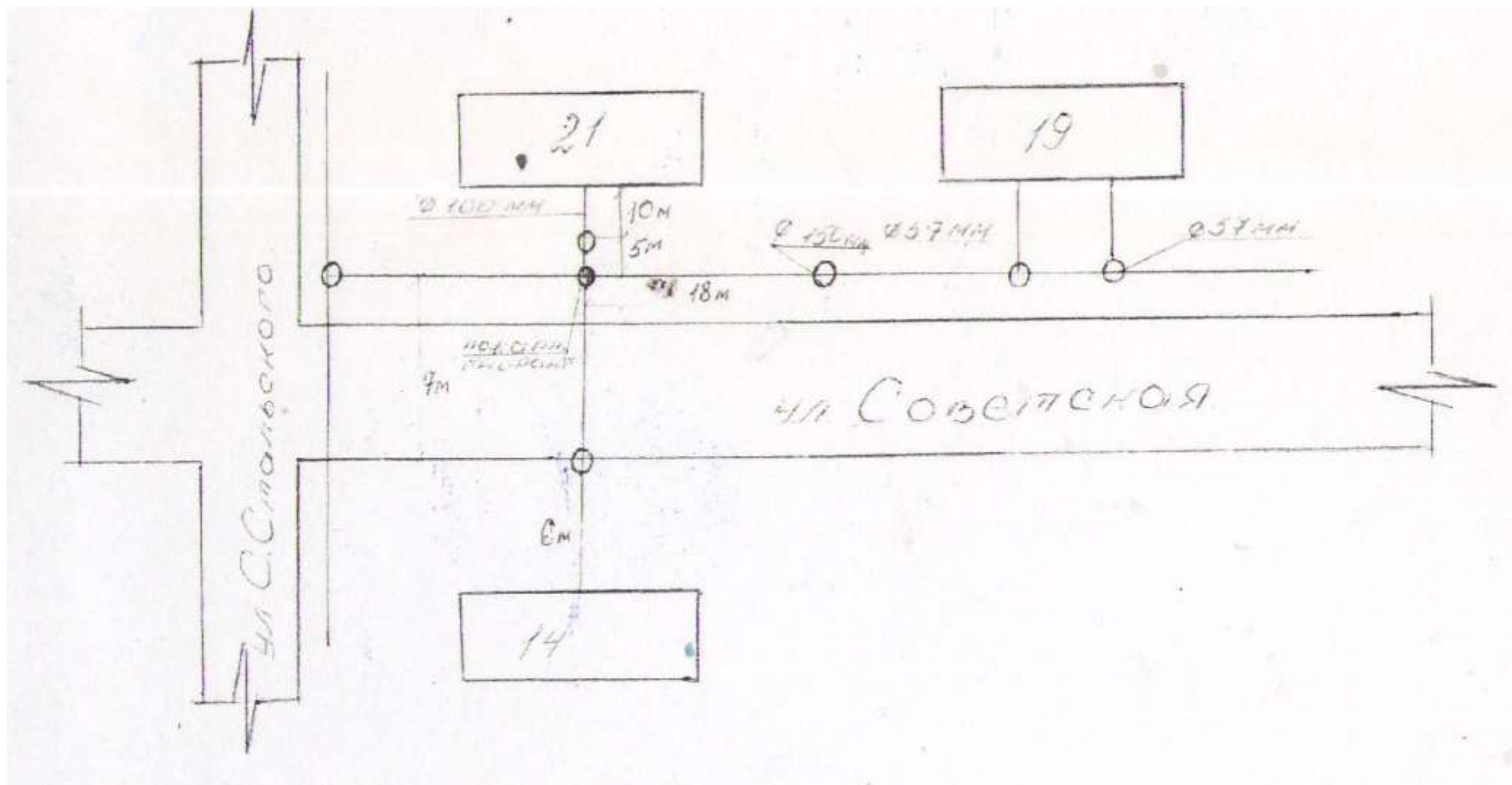
Схема водоснабжения улица Советская 21,19,14 21
