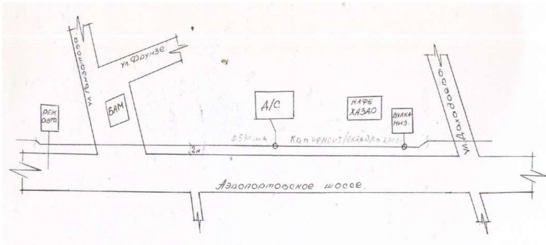
Схема водоснабжения Аэропортское шоссе
