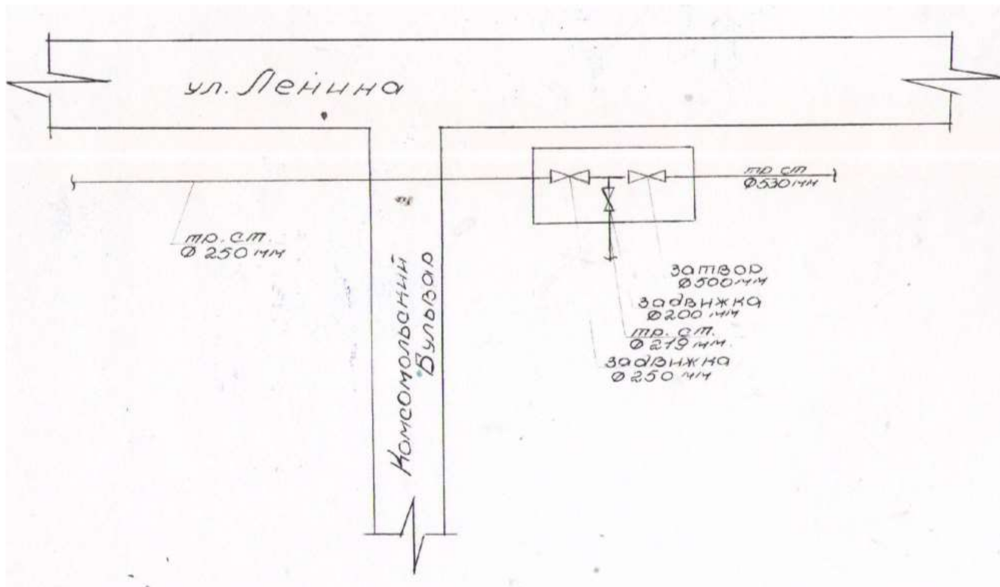
Схема водоснабжения улицы Ленина, Комсомольский бульвар узел колодца
