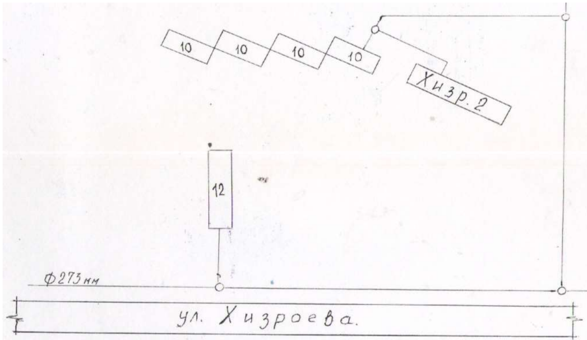
Схема водоснабжения Оржоникидзе 10,12, Хизроева 2
